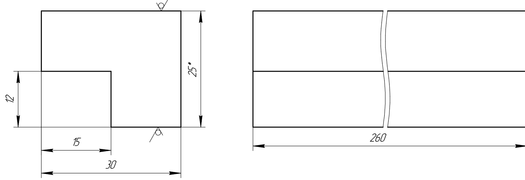
Дет. поз. 7 (2:1)
