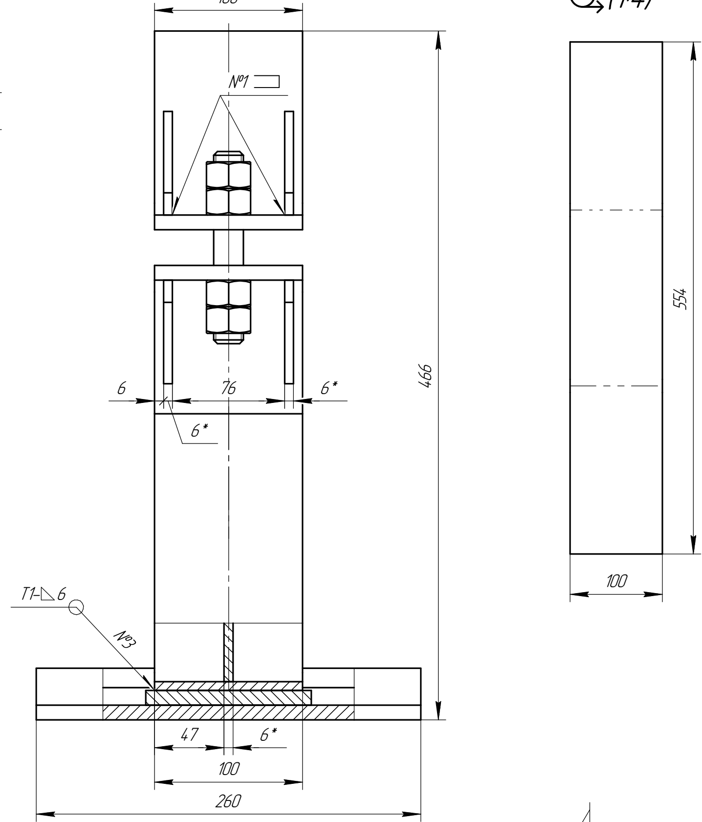
Дет. поз. 2
